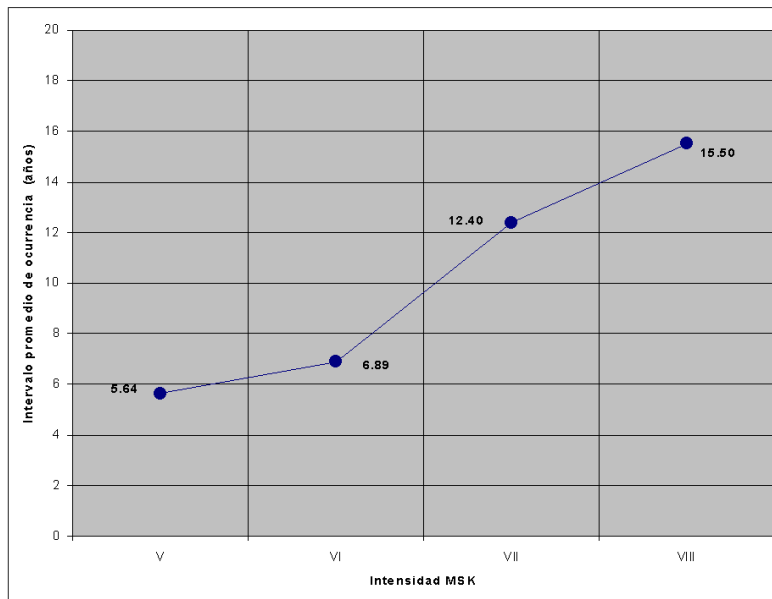
Gráfico N° 44. Recurrencias Ourrencia en Años, de Sismos Dañinos para la Región.
