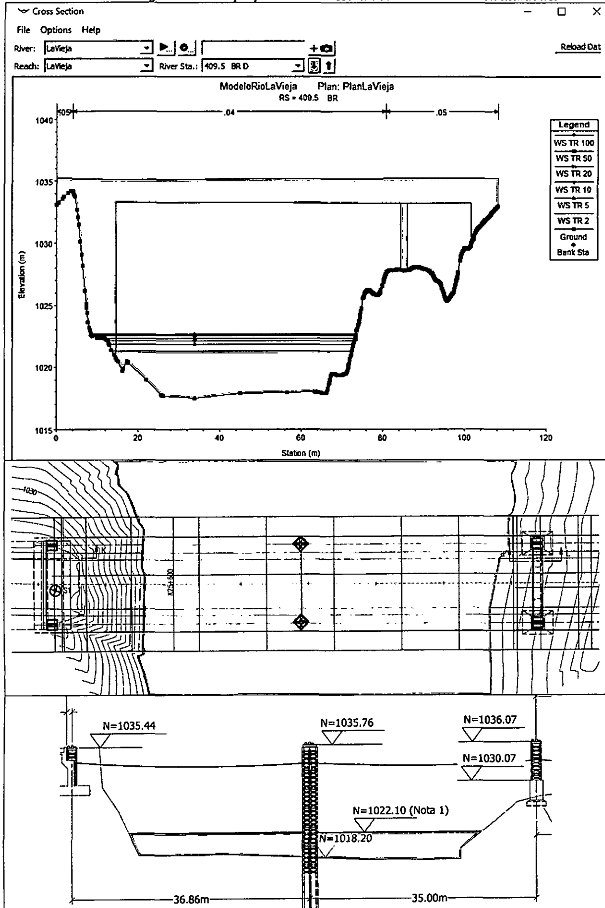
Figura 1. Obras propuestas con resultados de la modelación hidráulica
