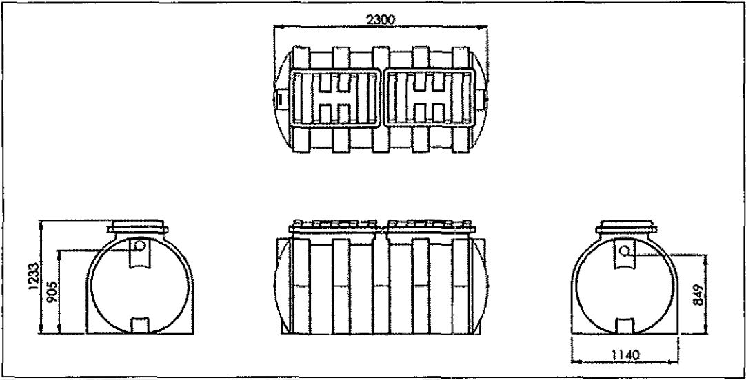
Imagen 4. Tanque séptico prefabricado integrado
