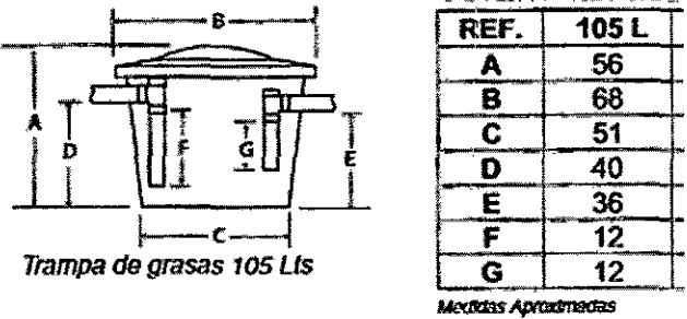
Imagen 3. Trampa de grasas prefabricada
