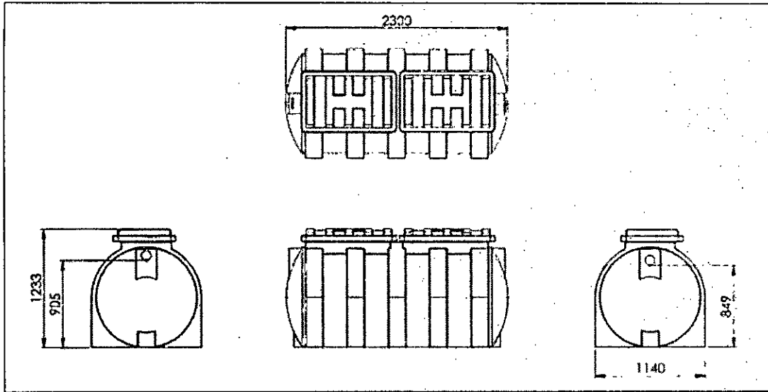
Imagen 2. Sistema de tratamiento integrado prefabricado
