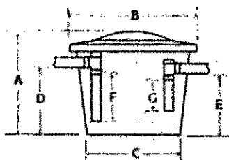
Trampa de grasas 105 Lts
