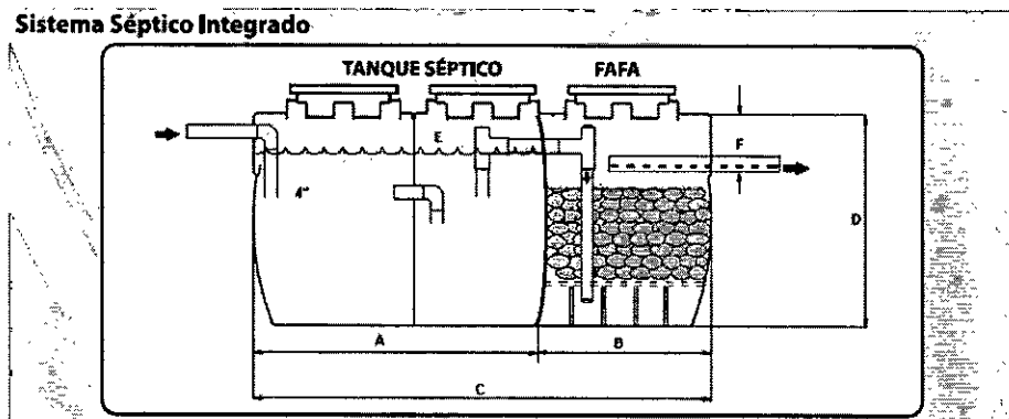
Imagen 1. Esquema corte de Tanque Séptico y FFA.
