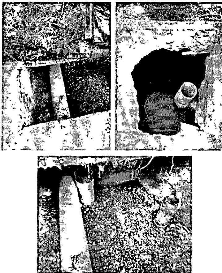
Imagen 4. Tubería que conecta del tanque séptico al pozo de absorción, y funcionamiento del FAFA.
