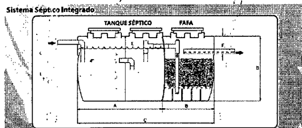
Imagen 1. Esquema corte de Tanque Séptico y FAFA.
