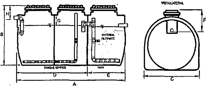
Imagen Ilustrativa N° 2. Sistema séptico integrado de 7500 ls capacidad
