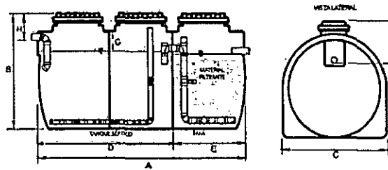
Imagen Ilustrativa N° 3. Sistema séptico integrado de 7500 lt. autolimpiable.
