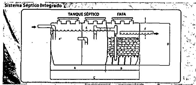
Imagen 1. Esquema corte de Tanque Séptico y FAFA.
