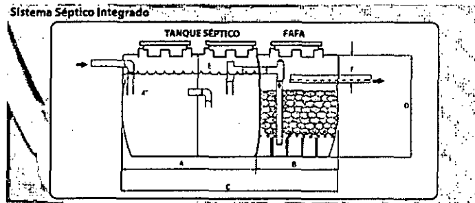
Imagen 1. Esquema corte de Tanque Séptico y FFA.
