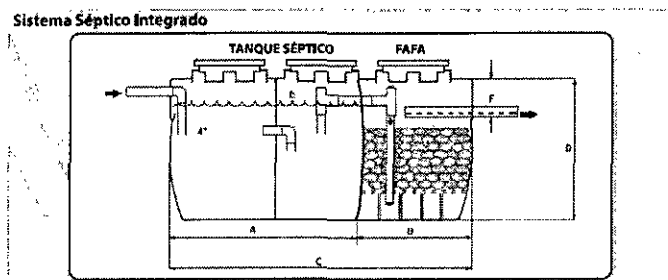
Imagen 1. Esquema corte de Tanque Séptico y FAFA.
