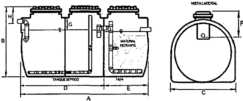
Imagen Ilustrativa N° 2, sistema séptico integrado de 7500 lts autolimpiable
