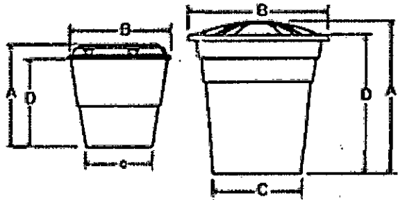
Tanque de 500Lts y 1000 Lts Tanque de 2000 Lts
