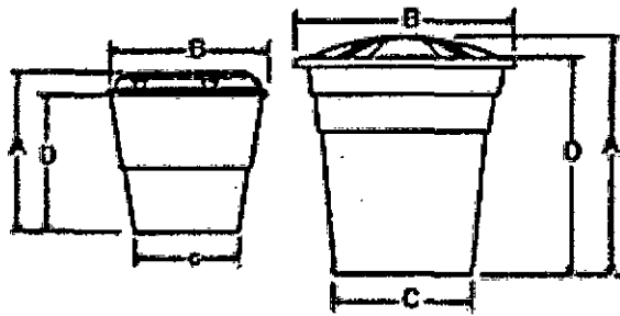
Tanque de 500Lts y 1000 Lts Tanque de 2000 Lts Dimensiones en metros [cm]
