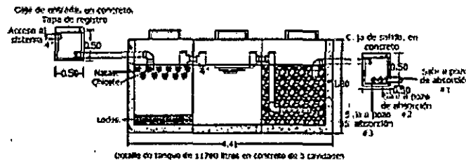
Imagen 1. Esquema corte de Tanque Séptico y FABA.
