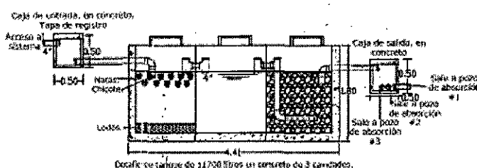
Imagen 1. Esquema corte de Tanque Séptico y FAFA.
