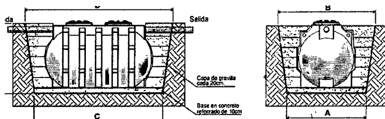
Imagen 1. Esquema corte de Tanque Séptico y FAFA.
