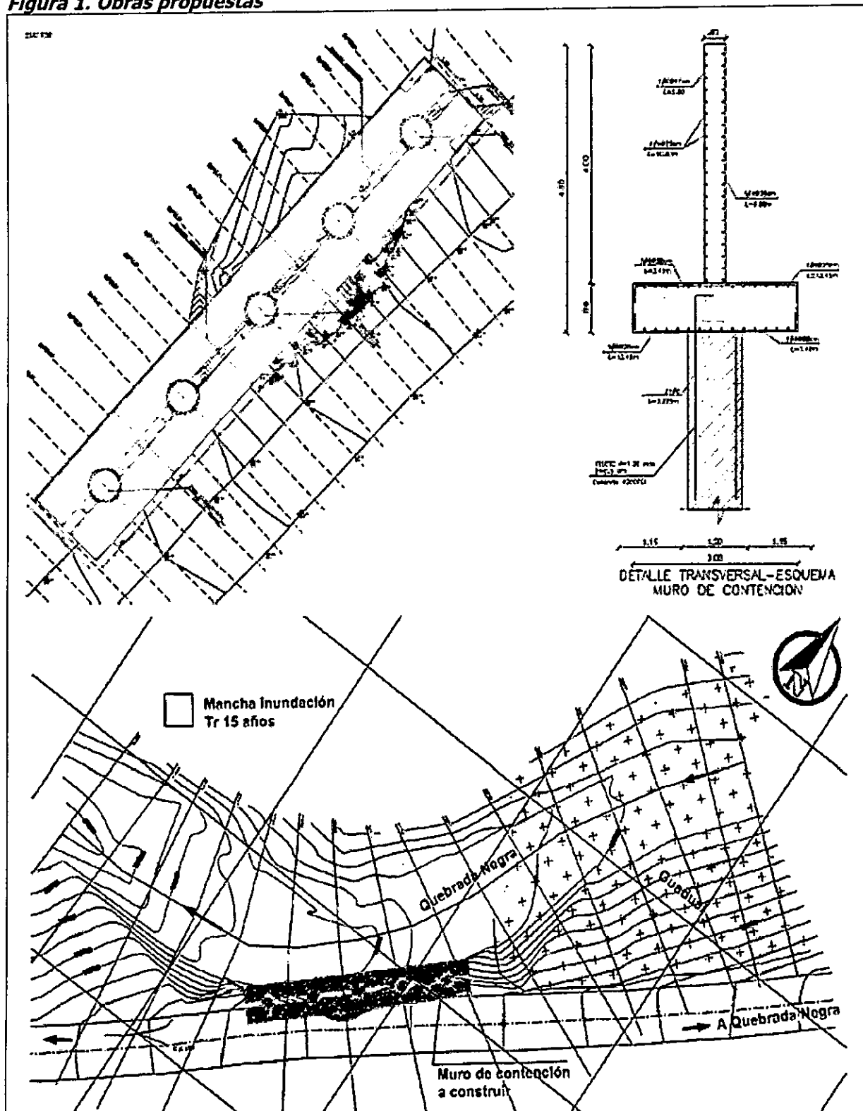
Figura 1. Obras propuestas
