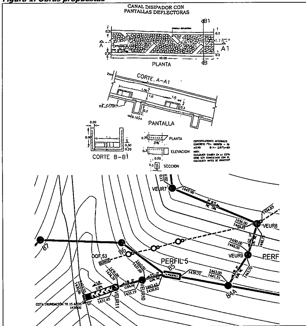
Figura 1. Obras propuestas
