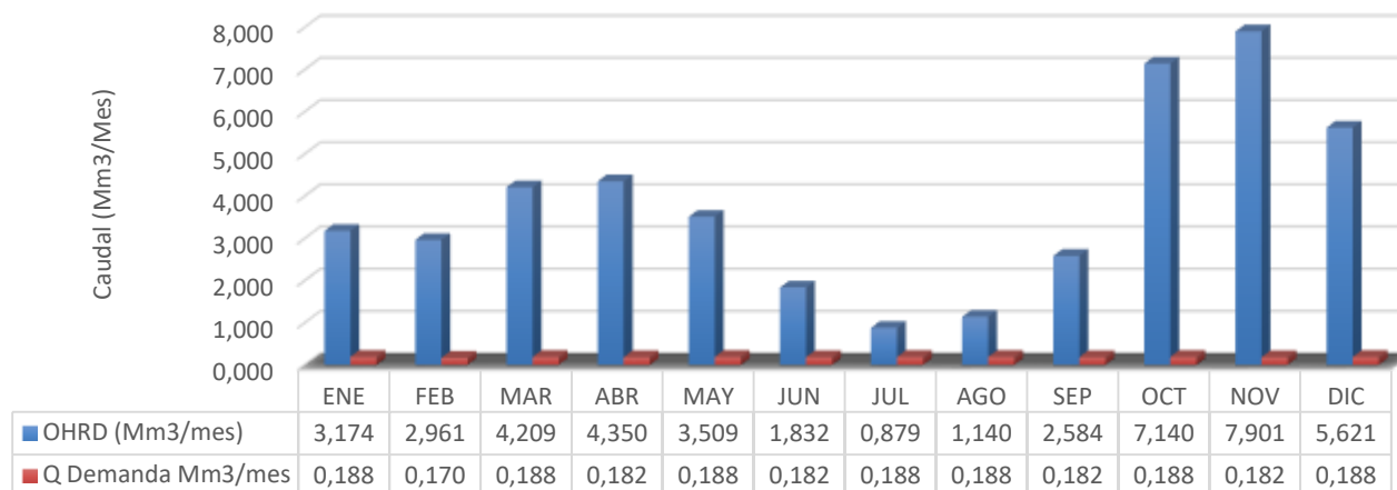
OFERTA Y DEMANDA HIDRICA (Mm3/Mes) RÍO BARBAS
