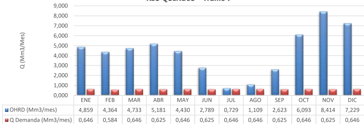
OFERTA Y DEMANDA HIDRICA (Mm³/mes) RIO QUINDIO - Tramo 7
