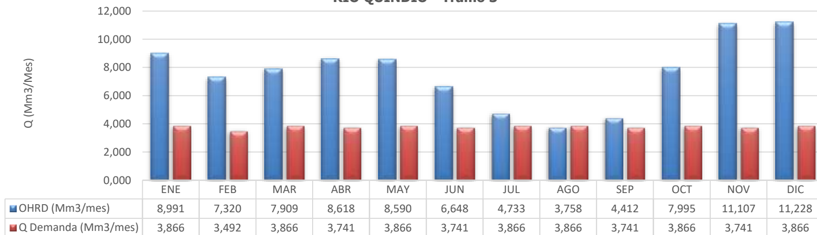
OFERTA Y DEMANDA HIDRICA (Mm 3 /mes) RIO QUINDIO - Tramo 3
