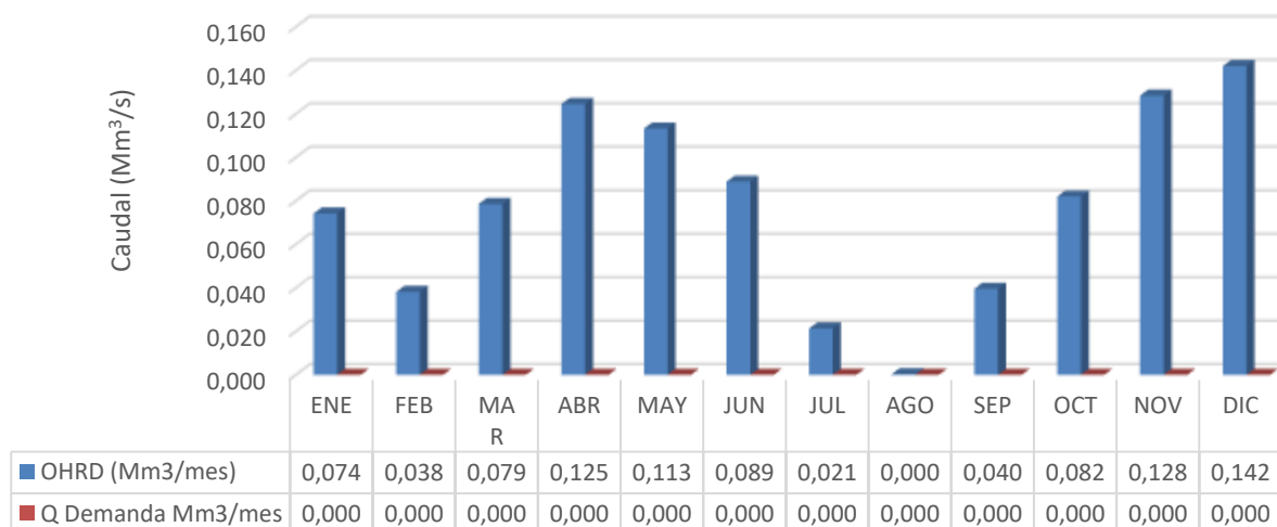
OFERTA Y DEMANDA HIDRICA (Mm 3 /mes) RÍO ROBLE TRAMO IV
