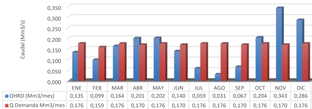
OFERTA Y DEMANDA HIDRICA (Mm 3 /mes) QUEBRADA LACHA
