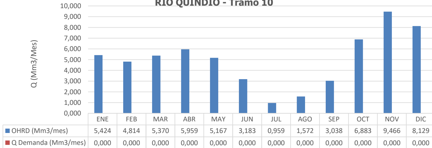
OFERTA Y DEMANDA HIDRICA (Mm 3 /mes) RIO QUINDIO - Tramo 10
