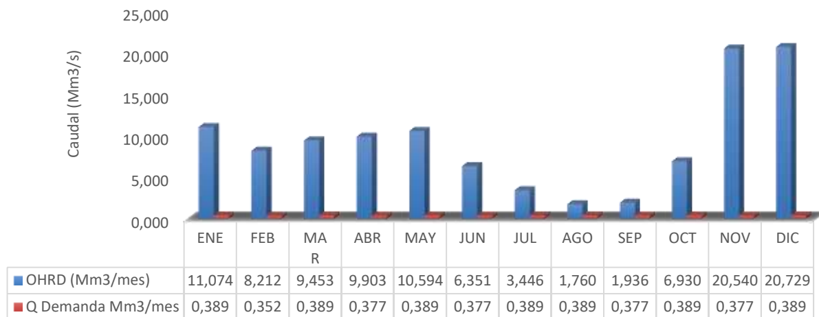
OFERTA Y DEMANDA HIDRICA (Mm 3 /Mes) RÍO LEJOS
