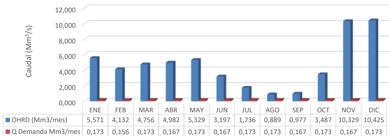
OFERTA Y DEMANDA HIDRICA (Mm 3 /mes) RÍO ROJO
