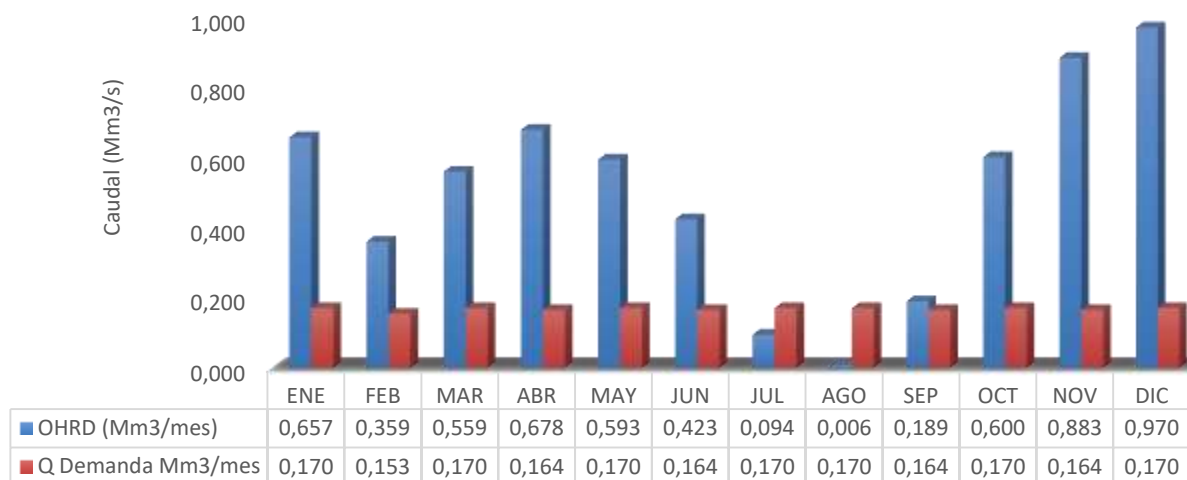
OFERTA Y DEMANDA HIDRICA (Mm 3 /mes) RÍO ROBLE TRAMO V
