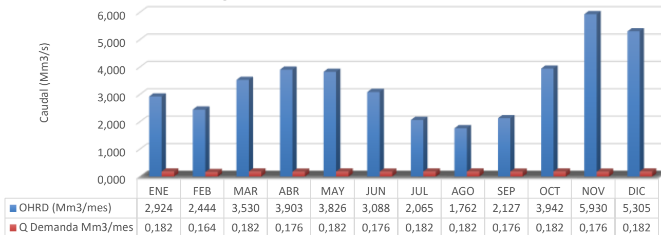
OFERTA Y DEMANDA HIDRICA (Mm3/mes) QUEBRADA BUENAVISTA TRAMO II
