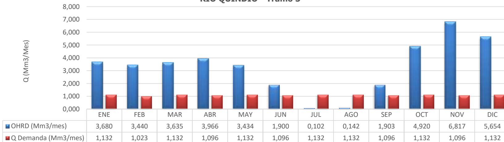
OFERTA Y DEMANDA HIDRICA (Mm3/mes) RIO QUINDIO - Tramo 5
