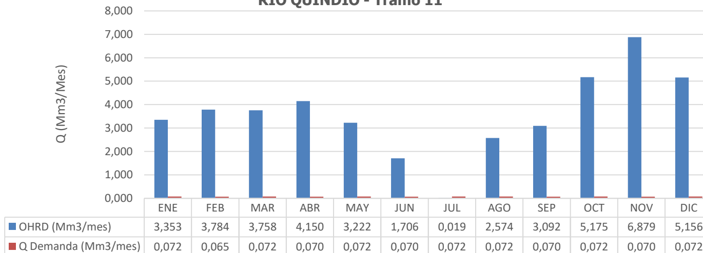
OFERTA Y DEMANDA HIDRICA (Mm 3 /mes) RIO QUINDIO - Tramo 11
