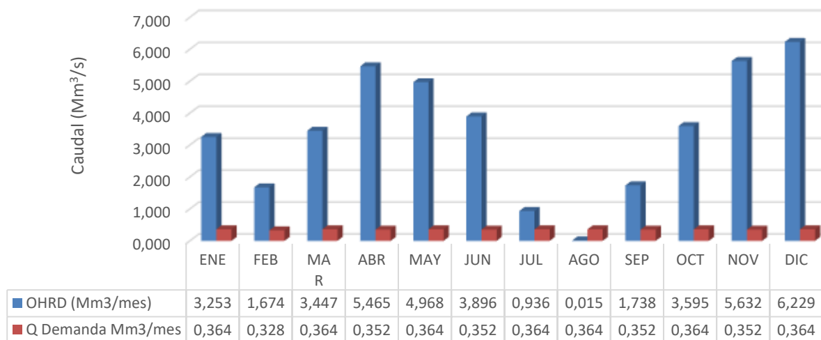
OFERTA Y DEMANDA HIDRICA (Mm 3 /mes) RÍO ROBLE TRAMO VII
