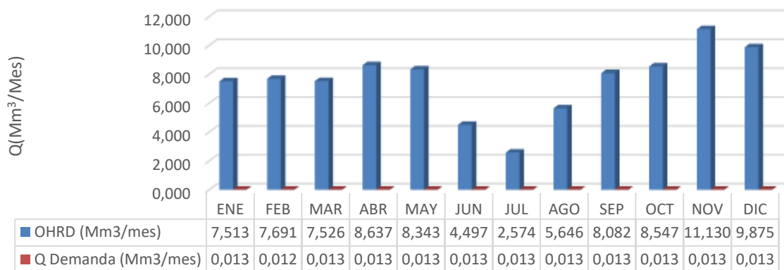
OFERTA Y DEMANDA HIDRICA (Mm 3 /mes) RIO QUINDIO - Tramo 12
