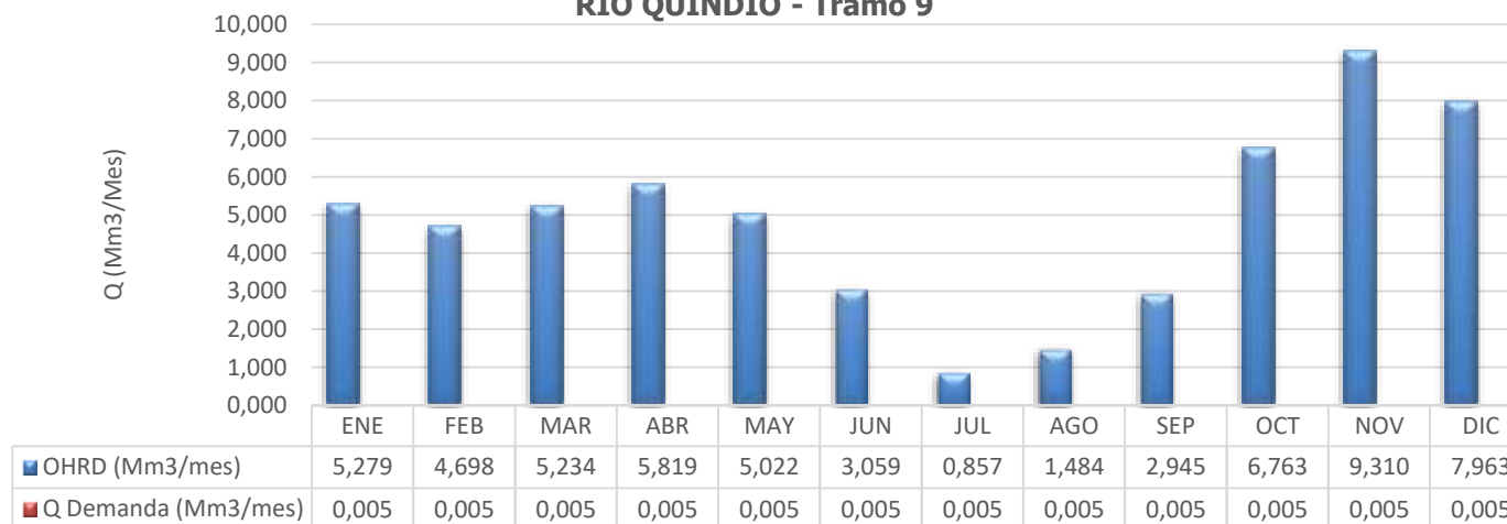
OFERTA Y DEMANDA HIDRICA (Mm 3 /mes) RIO QUINDIO - Tramo 9
