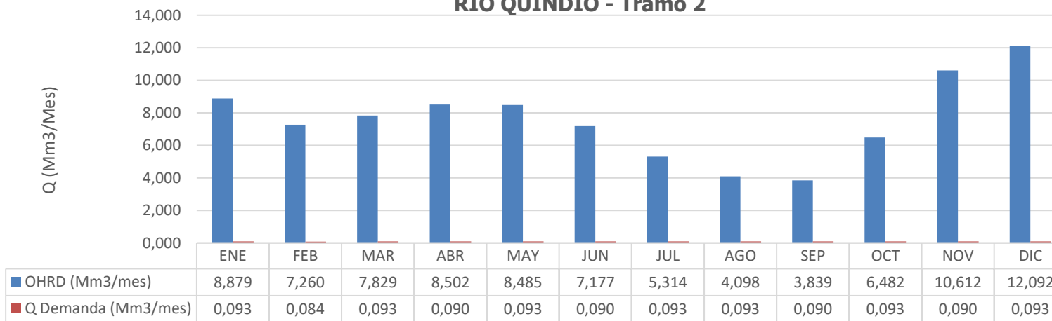
OFERTA Y DEMANDA HIDRICA (Mm 3 /mes) RIO QUINDIO - Tramo 2
