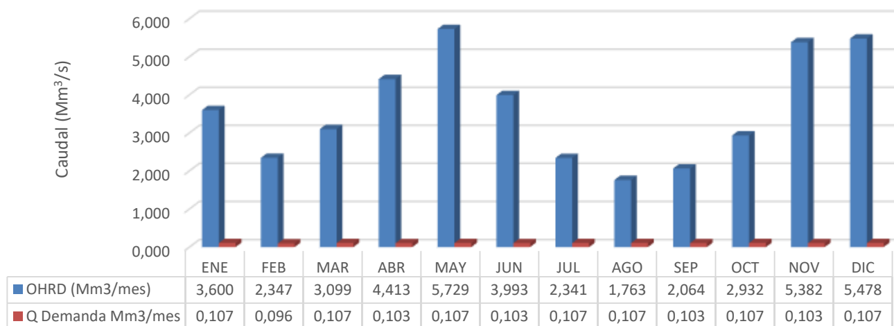
OFERTA Y DEMANDA HIDRICA (Mm 3 /mes) RÍO ESPEJO
