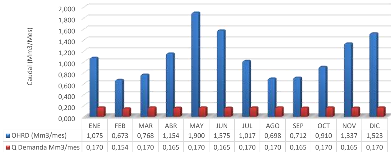
OFERTA Y DEMANDA HIDRICA (Mm 3 /Mes) QUEBRADA CRISTALES
