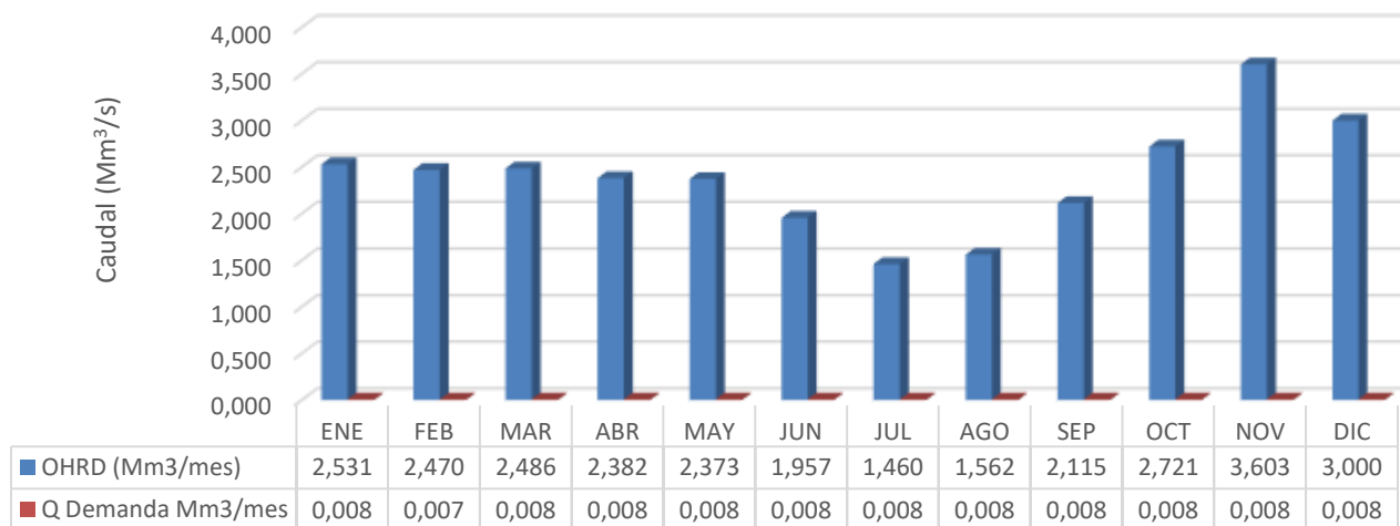
OFERTA Y DEMANDA HIDRICA (Mm 3 /mes) RÍO NAVARCO
