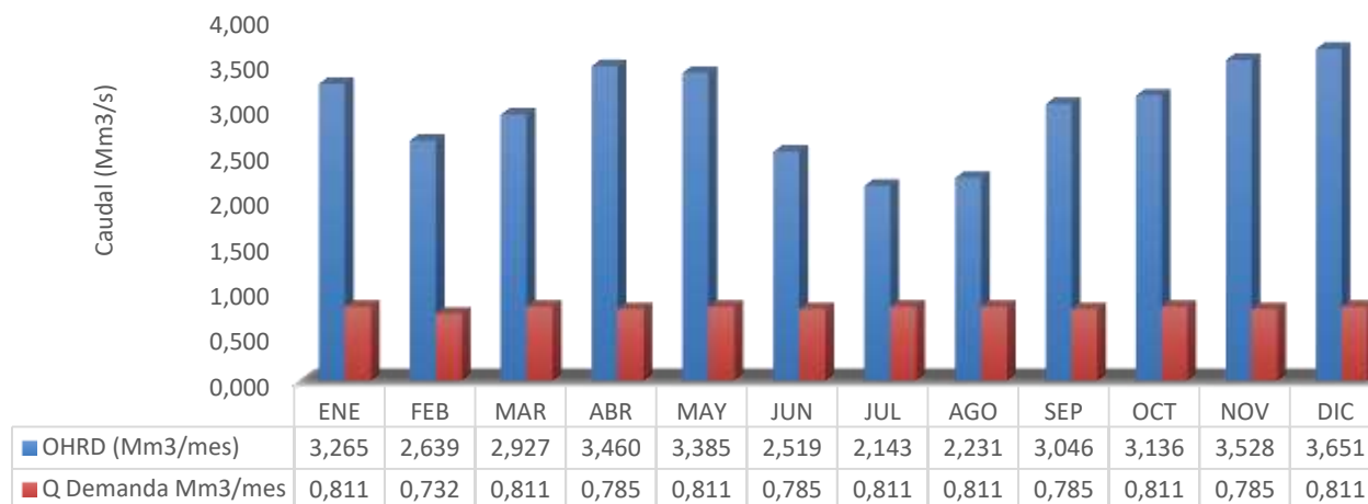
OFERTA Y DEMANDA HIDRICA (Mm 3 /mes) RÍO SANTO DOMINGO
