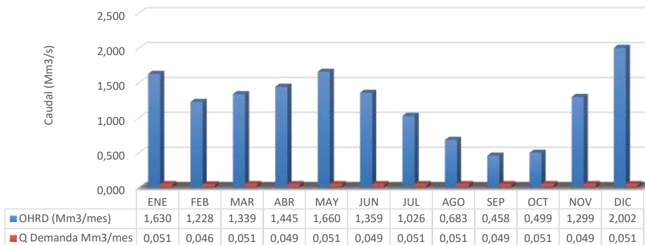
OFERTA Y DEMANDA HIDRICA (Mm 3 /mes) QUEBRADA LA PICOTA
