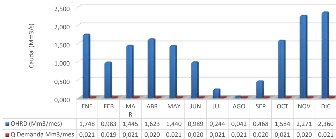
OFERTA Y DEMANDA HIDRICA (Mm 3 /mes) RÍO ROBLE TRAMO II
