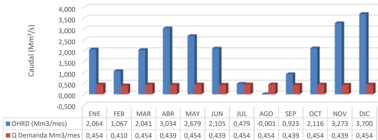
OFERTA Y DEMANDA HIDRICA (Mm 3 /mes) RÍO ROBLE TRAMO VI
