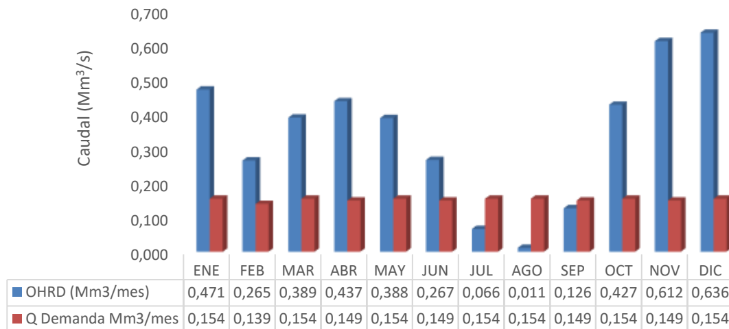
OFERTA Y DEMANDA HIDRICA (Mm 3 /mes) RÍO ROBLE TRAMO I
