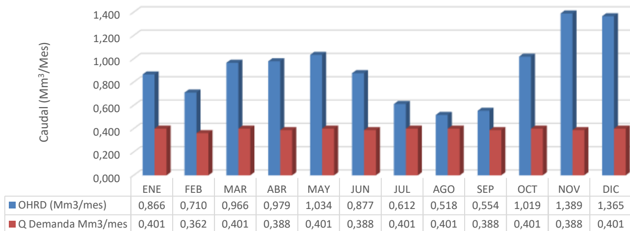
OFERTA Y DEMANDA HIDRICA (Mm 3 /Mes) QUEBRADA BUENAVISTA TRAMO I
