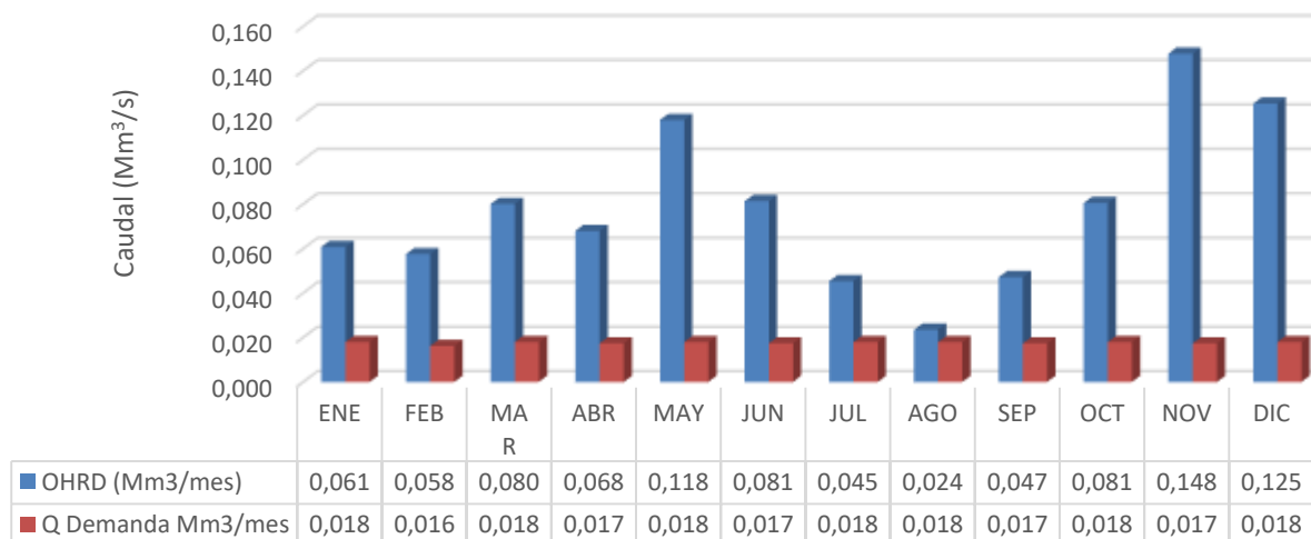
OFERTA Y DEMANDA HIDRICA (Mm 3 /mes) RÍO ROBLE TRAMO III
