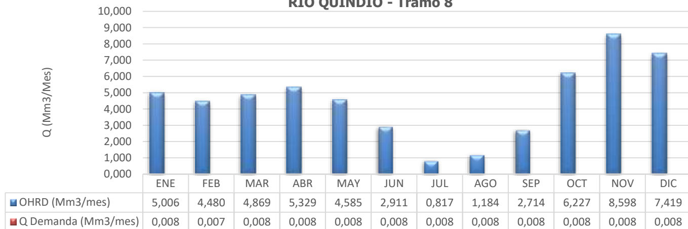
OFERTA Y DEMANDA HIDRICA (Mm 3 /mes) RIO QUINDIO - Tramo 8
