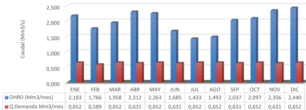
OFERTA Y DEMANDA HIDRICA (Mm 3 /mes) RÍO VERDE
