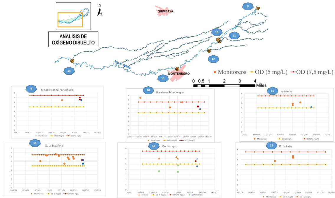
Figura 125. Variación de Oxígeno Disuelto en la Cuenca Baja del río Roble.
