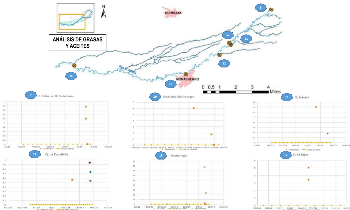
Figura 138. Variación de Grasas y Aceites en la Cuenca Alta y Media del río Roble.
