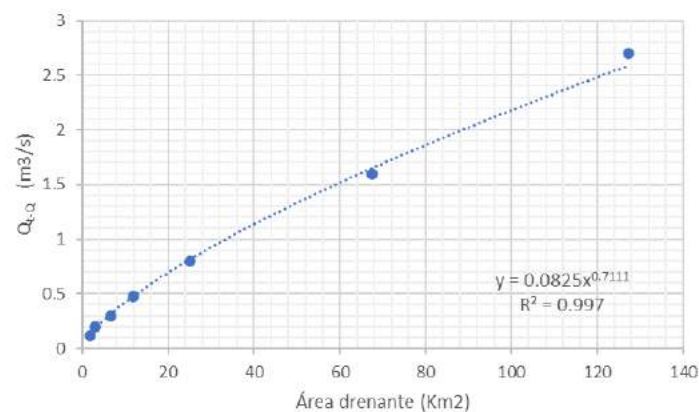
Figura 64. Caudal Q_{t-Q} en función del área de cuenca drenante a cada tramo en el río Roble, quebrada Portachuelo y quebrada Cajones.
