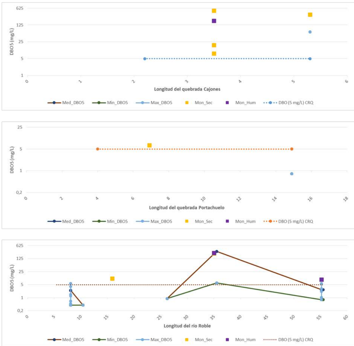
Figura 141. Valores Máximo, Mínimo y Medio de DBO5 en el río Roble, quebrada Cajones y quebrada Portachuelo.
