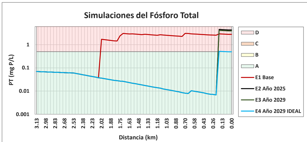
Figura 258. Resultados de las Simulaciones del Fósforo Total en la quebrada Cajones
