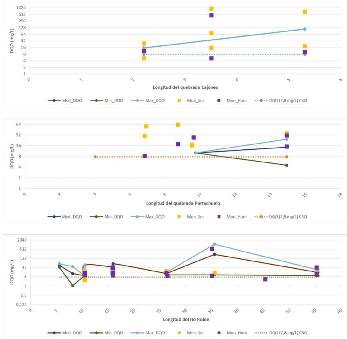
Figura 142. Valores Máximo, Mínimo y Medio de DQO en el río Roble, Quebrada Cajones y Quebrada Portachuelo.
