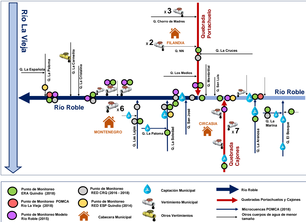
Figura 118. Topología de la red de drenaje del río Roble. Puntos de monitoreo POMCA (2018), ERA (2017), Modelo de calidad del agua (2015) y RED de Calidad CRQ (2014-2018)
