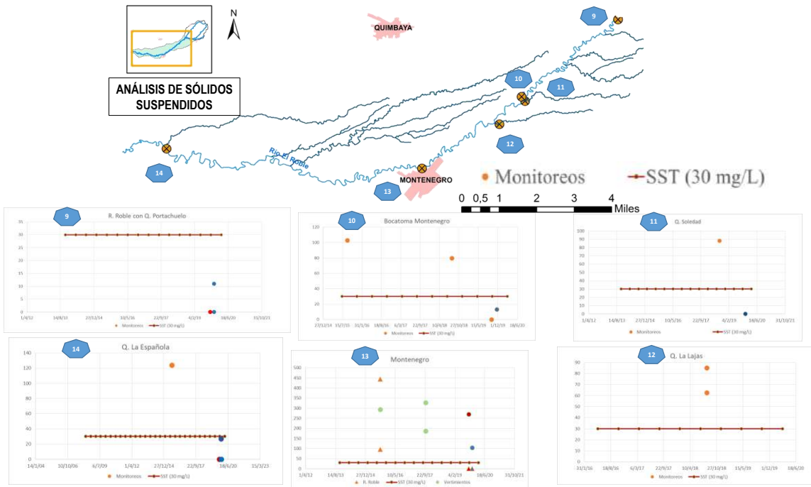
Figura 137. Variación de Sólidos Suspendidos Totales en la Cuenca Baja del río Roble.
