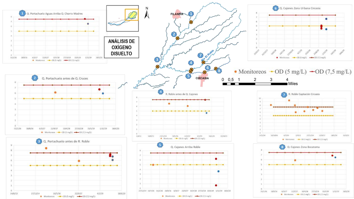
Figura 124. Variación de Oxígeno Disuelto en la Cuenca Alta y Media del río Roble.
