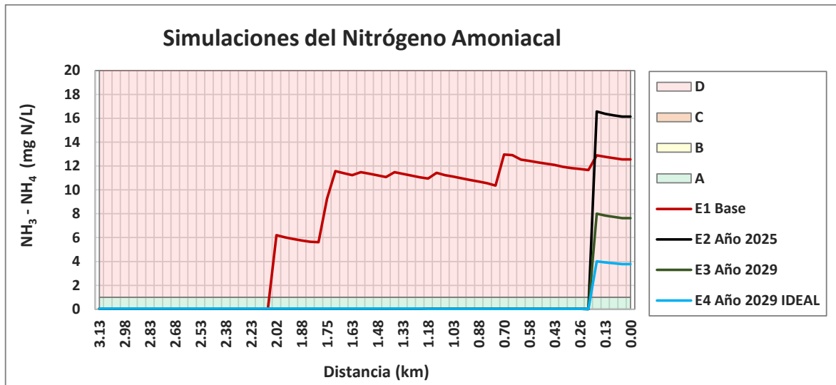
Figura 256. Resultados de las Simulaciones el Nitrógeno Amoniacal en la quebrada Cajones
