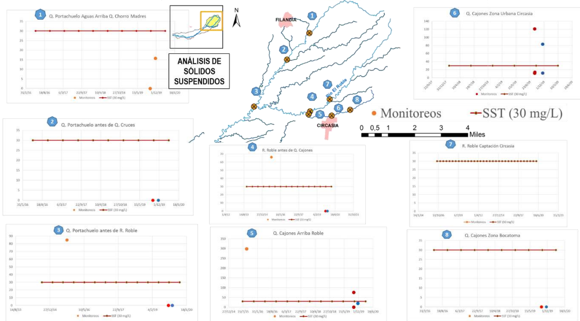
Figura 136. Variación de Sólidos Suspendidos Totales en la Cuenca Alta y Media del río Roble.
