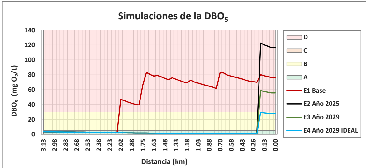
Figura 252. Resultados de las Simulaciones para la DBO 5 en la quebrada Cajones
